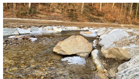
Einbau von sogenannten Störsteinen im Bachgerinne um auch bei Niederwasserführung unterschiedliche Wassertiefen- und Breiten zu erzeugen.
